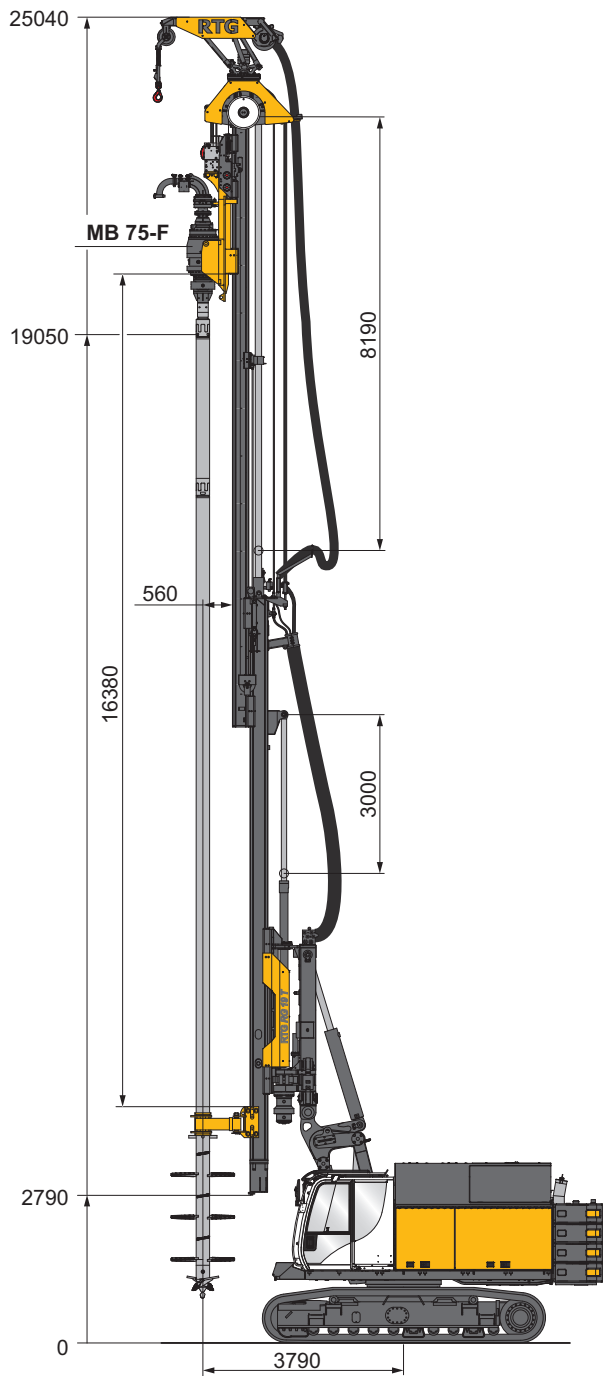
単軸ソイルミキシング SCM mixing
